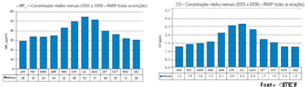
Figura 1 – Concentrações médias de MP 10 e CO
