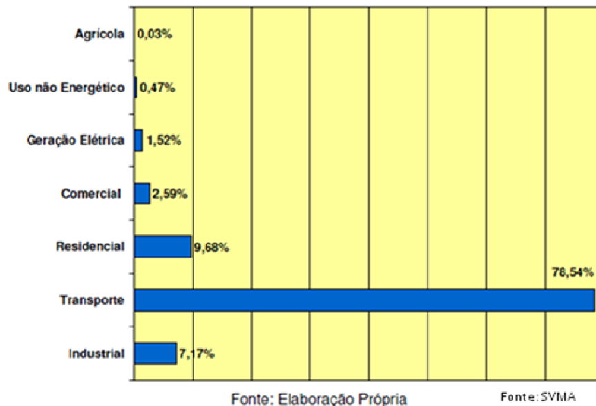
Figura 6 - Contribuição dos Setores Sócio-Econômicos nas Emissões do Uso de Energia pelo Município de São Paulo, em 2003 (%).
