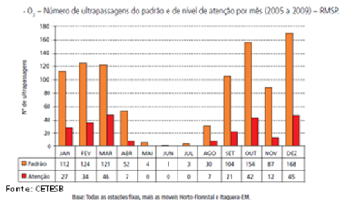
Figura 2 - Ultrapassagens do padrão e atenção por ozônio
