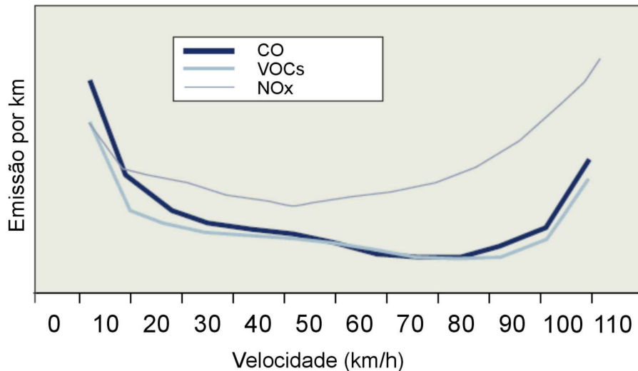
Figura 10 - Influência da velocidade sobre as emissões de veículos leves
