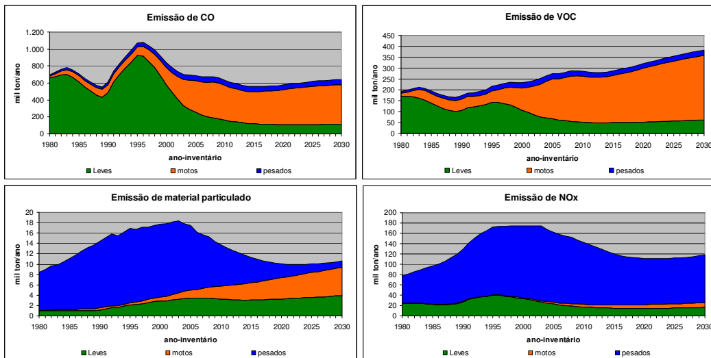
Figura 5 – Evolução das emissões dos principais poluentes locais na RMSP
