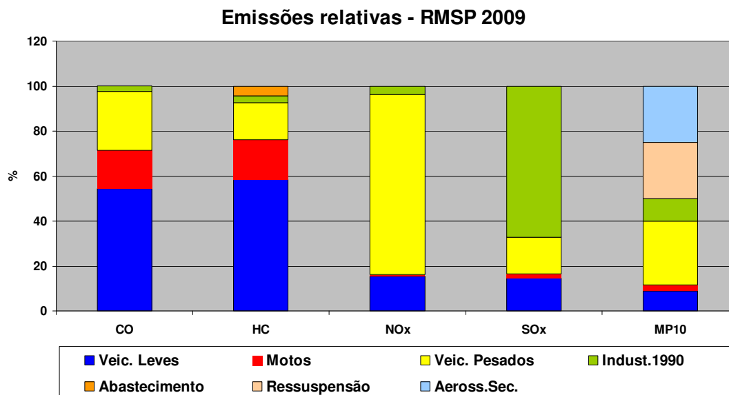
Figura 4 - Contribuição relativa das fontes de emissão na RMSP em 2009
